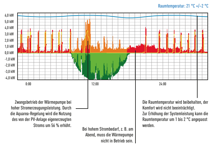
Typisches Profil für Stromverbrauch und -erzeugung mit Aquarea-Regelung
