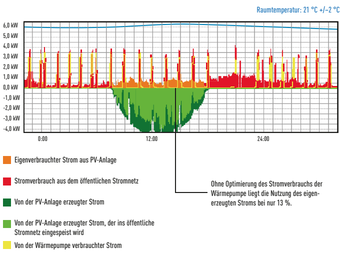
Typisches Profil für Stromverbrauch und -erzeugung ohne Aquarea-Regelung
