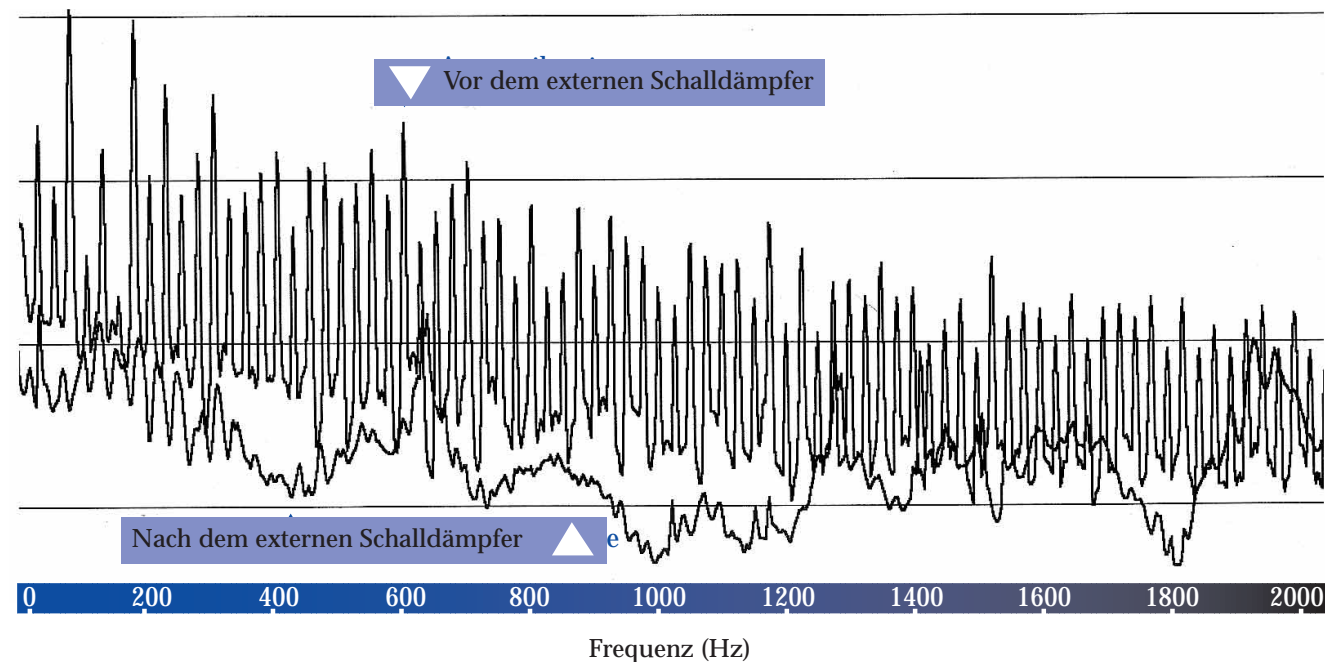
GEGLÄTTETE VERDICHTUNGSGAS-PULSATIONEN: dB
