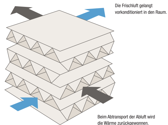
Die Struktur des Papierkreuzwärmetauschers
